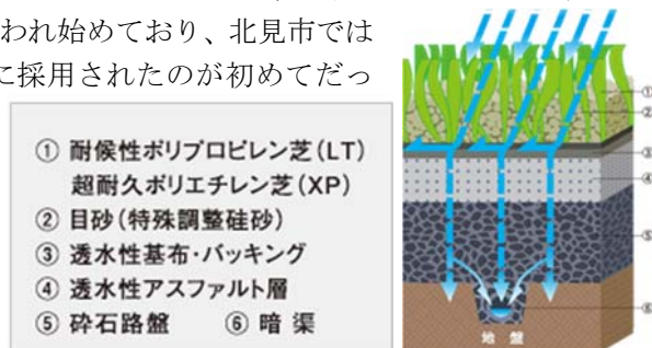
オムニコートの構造 (住友ゴムHPより)
